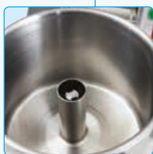
Tubo vasca rialzato per massimizzare la capacità effettiva di liquidi
